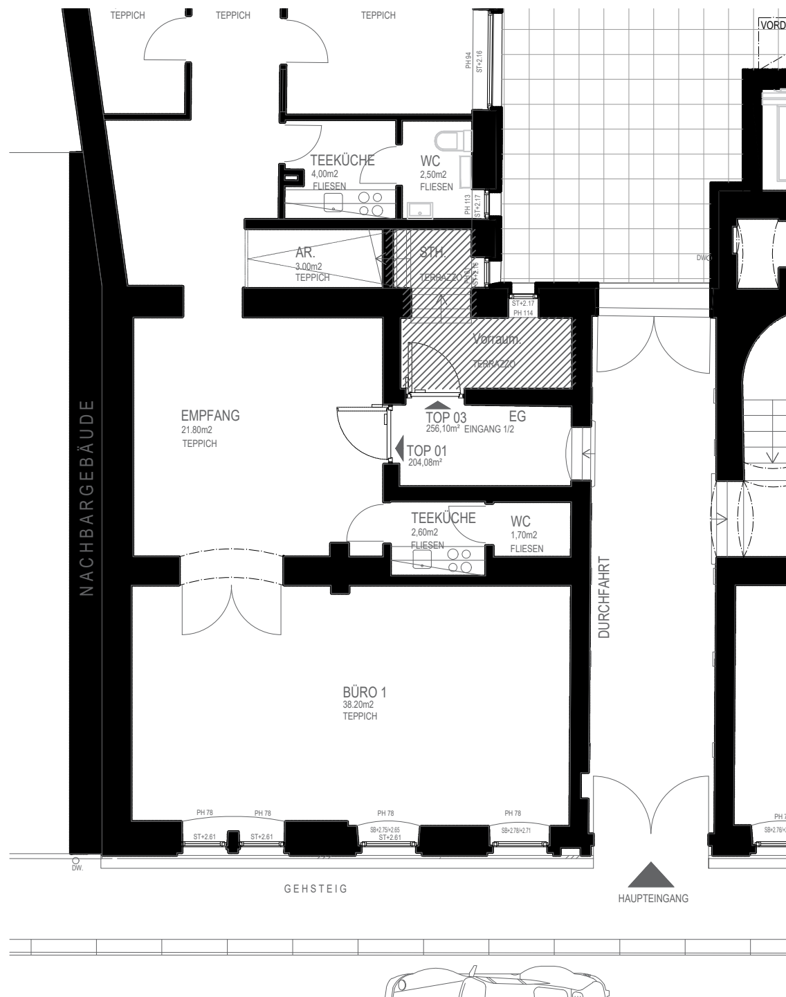
STRASSENANSICHT
