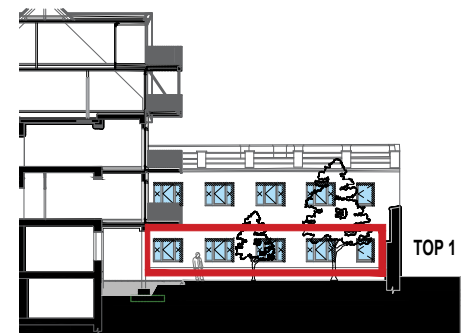
INNENHOFANSICHT
